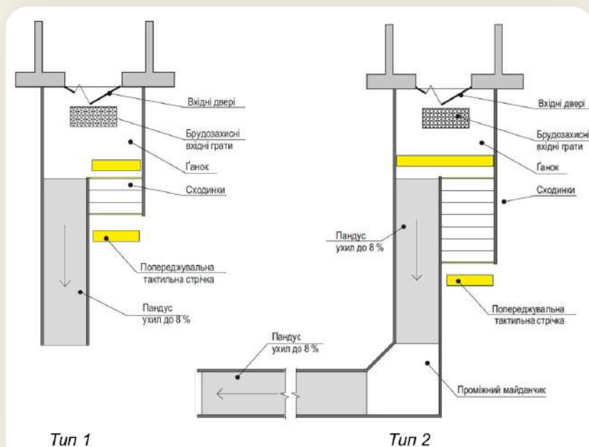
Рисунок 1.23.1. Типи облаштування вхідної групи: а – прямий пандус; б, в – кутовий пандус розміщений вздовж тротуару
