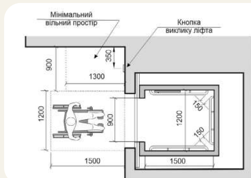
Рисунок 1.43. Схема доступного ліфта
