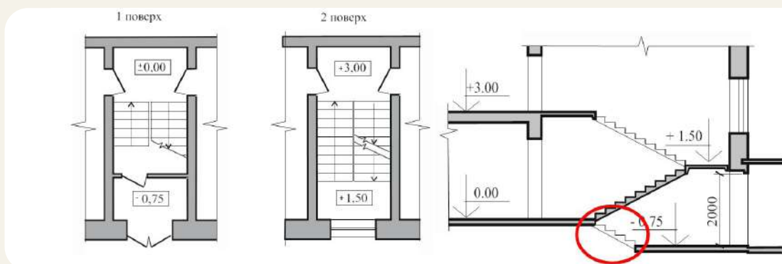
Рисунок 1.36. Сходинок цокольного поверху типове рішення
