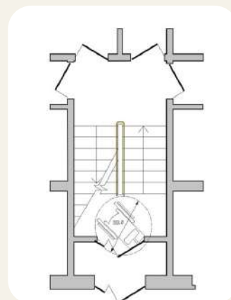
Рисунок 1.34. Схема забезпечення доступності до сходинок на цокольному поверсі
