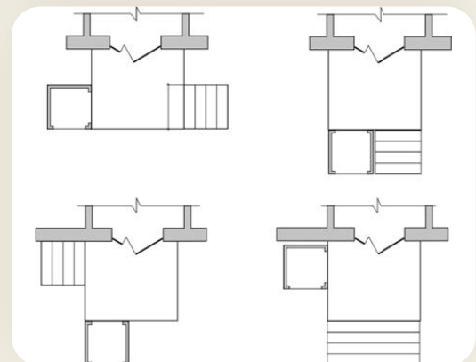
Рисунок 1.27. Взаємне розміщення підймальних пристроїв і сходів
