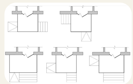
Рисунок 1.20. Рекомендовані схеми взаємного розміщення пандуса і сходів
