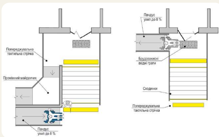
Рисунок 1.21. Неприпустиме взаємне розміщення пандуса і сходів
