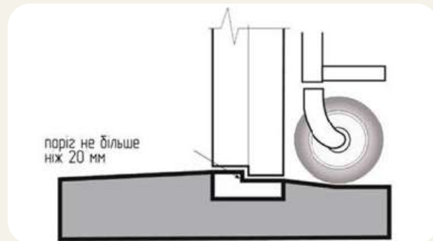
Рисунок 1.9. Порог вхідного вузла
