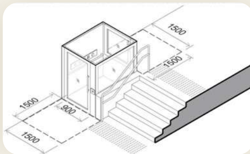
Рисунок 1.42. Приклад влаштування підйомального пристрою з вертикальним переміщенням кабіни.
