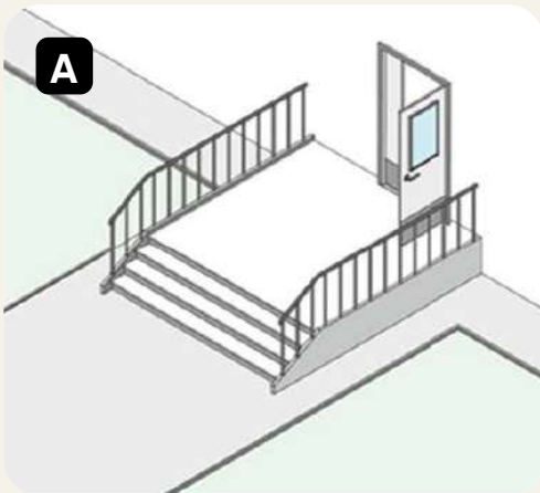
Рисунок 1.25. Варіанти влаштування пандуса для ґанків висотою до 75 см:
