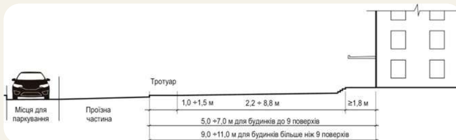
Рисунок 1.3. Облаштування доступного безбар'єрного входу в будинок в разі 1 або 2 сходинок ґанку:
