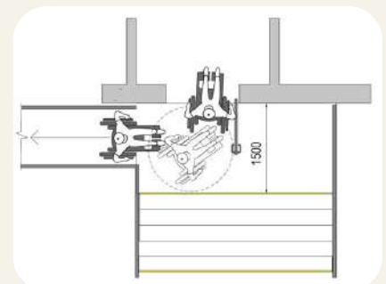
Рисунок 1.22. Схема маневру- вання кріслом колісним на ганку
