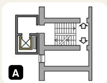
Рисунок 1.30. Прибудова ліфта до сходової клітки: а – 1 поверх наявний стан; б – 1 поверх з прибудовою ліфта; с – типовий поверх
