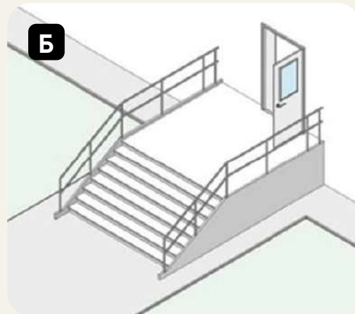
Рисунок 1.24. Приклад наявних ґанків:
