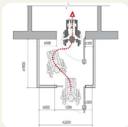
Рисунок 1.35. Схема маневрування в межах тамбура
