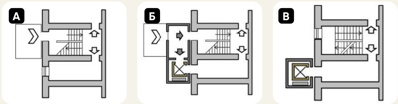
Рисунок 1.30. Прибудова ліфта до сходової клітки: а – 1 поверх наявний стан; б – 1 поверх з прибудовою ліфта; с – типовий поверх
