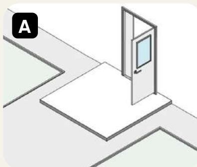
Рисунок 1.3. Облаштування доступного безбар'єрного входу в будинок в разі 1 або 2 сходинок ґанку:
