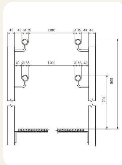
Рисунок 1.17. схема розрізу пандуса
