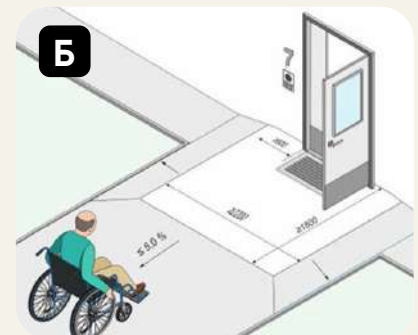
Рисунок 1.4. Приклади забезпечення входу в будинок з рівня вимощення Вхідні двері
