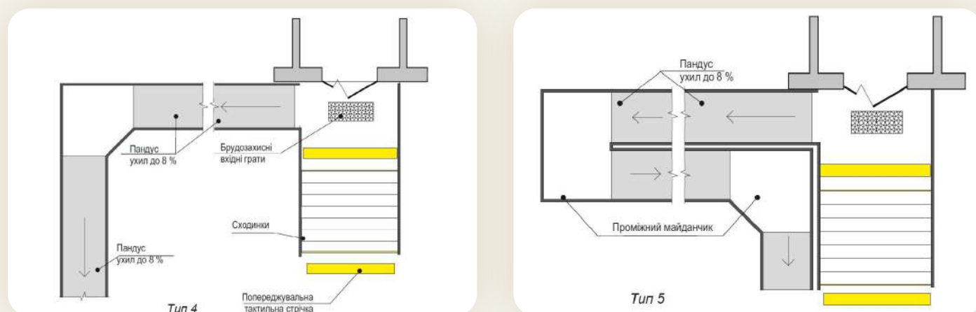
Рисунок 1.23.3. Типи облаштування вхідної групи (продовження): д) П-подібний пандус
