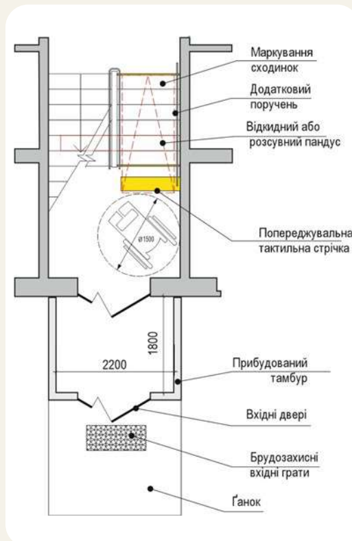
Рисунок 1.38. Схема адаптації входів до першого поверху в будинках типових серій
