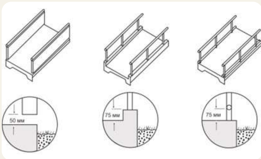
Рисунок 1.16. Облаштування поздовжніх країв пандуса
